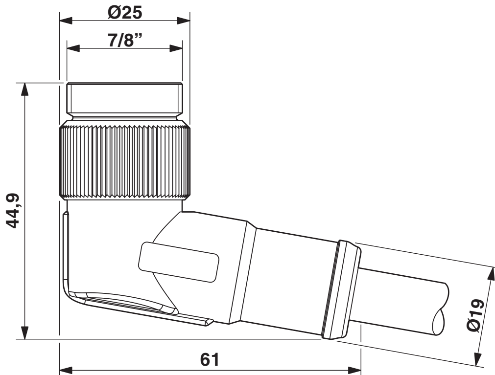
Connettore maschio 7/8"-16UNF, angolato
