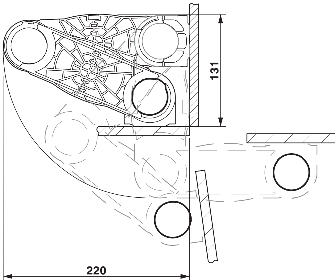
Dessin coté
