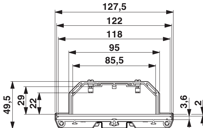
Dessin coté
