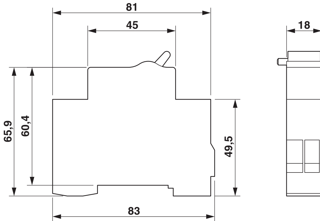
Dessin coté
