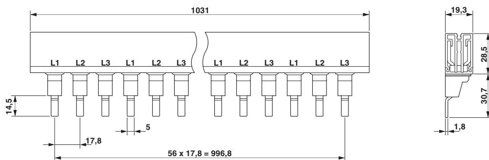
Dessin coté
