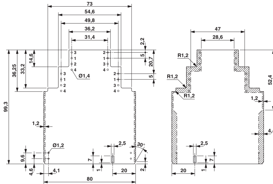
Dessin coté des circuits imprimés ME... pour l'utilisation du capot à deux étages
