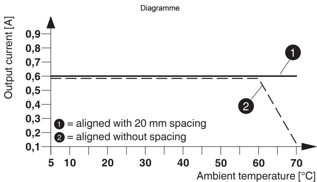
Courbe de capacité de charge
