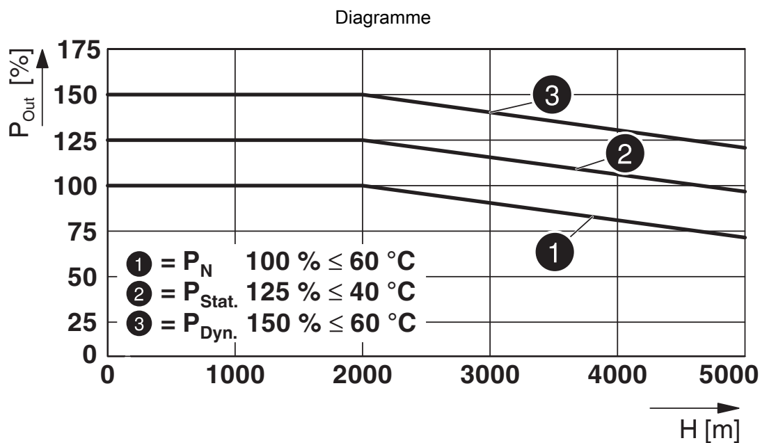
Puissance de sortie en fonction de la hauteur d'installation
