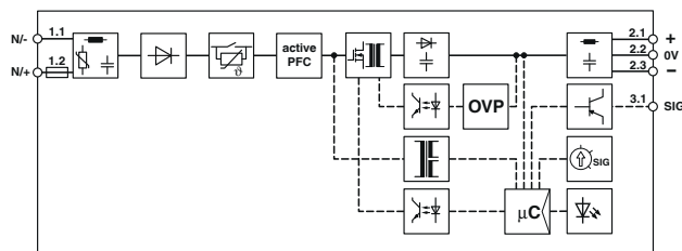
Schéma fonctionnel
