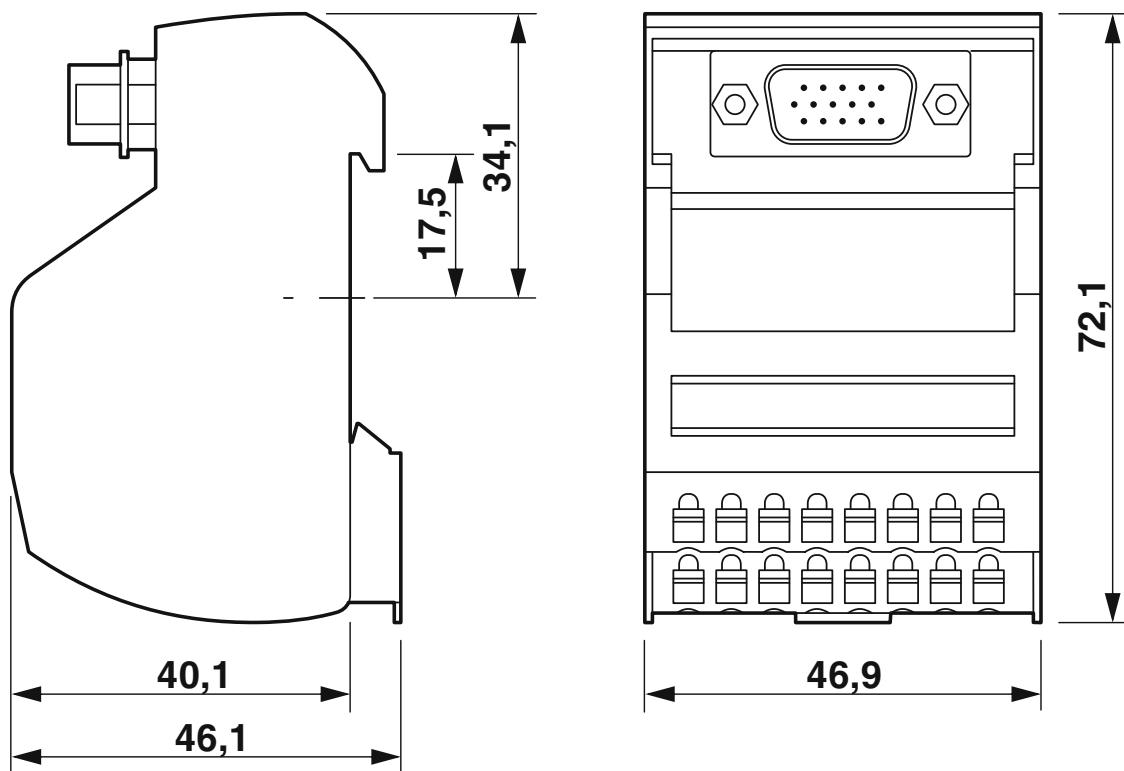
Dessin coté
