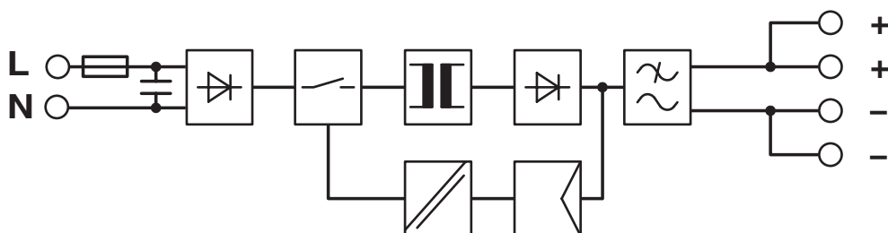
Schéma fonctionnel
