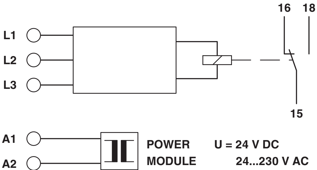
Schéma fonctionnel
