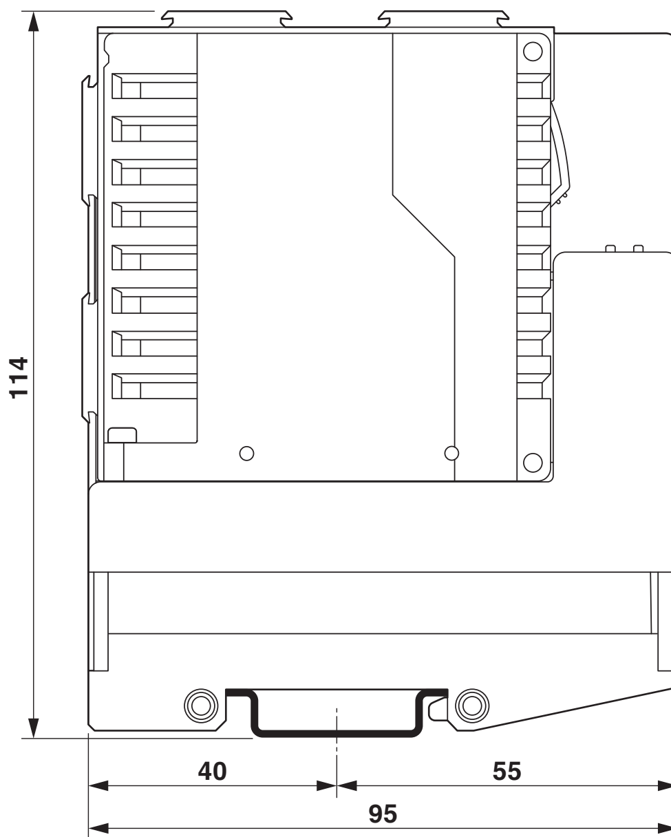
Dessin coté
