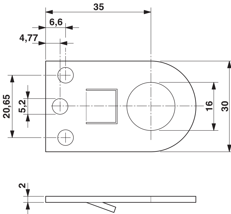
Dessin coté
