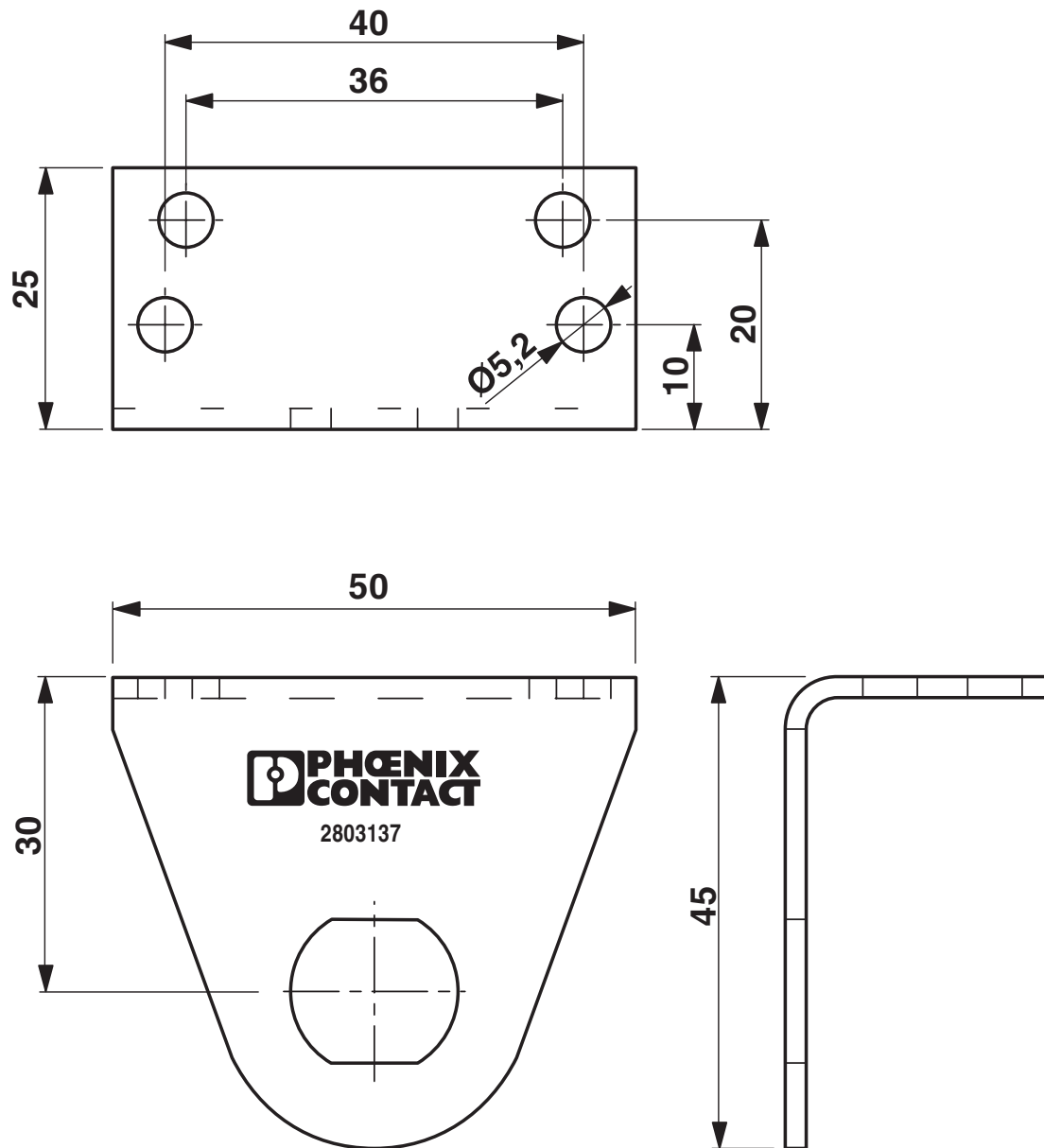
Dessin coté
