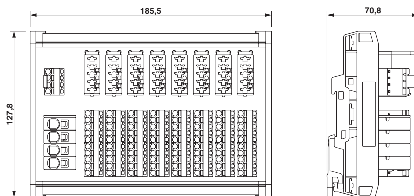
Dessin coté
