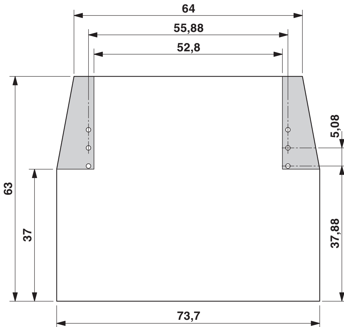
Dessin coté
