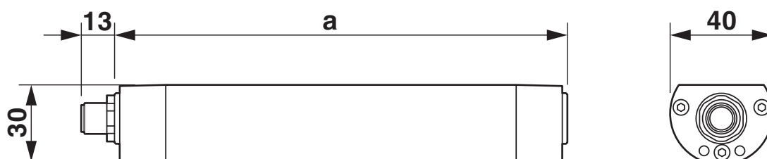
Dessin coté
