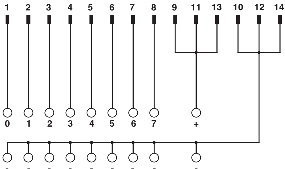
Schéma des connexions VIP-2/.../FLK14/8M/PLC
