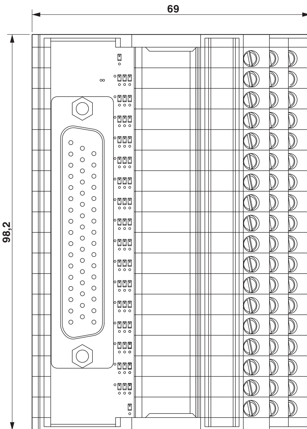
Dessin coté
