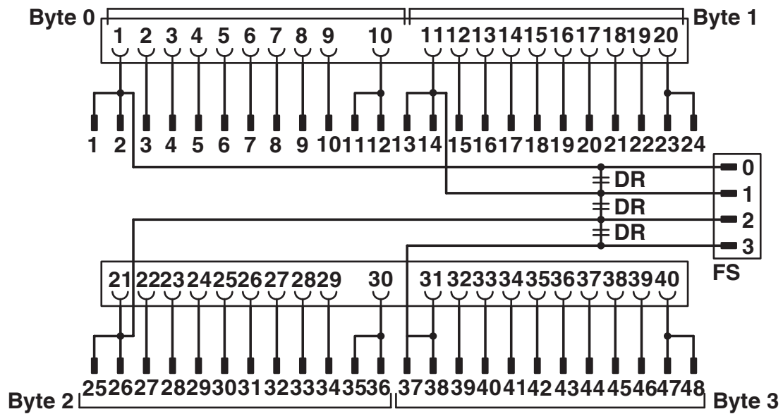
Schéma des connexions FLKM 50-PA-S300
