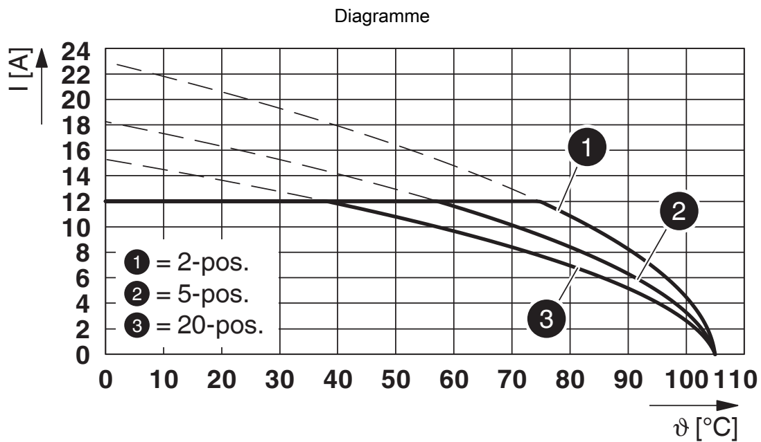
Type : FKCS 2,5/...-ST-5,08 avec MSTBV 2,5/...-G-5,08
