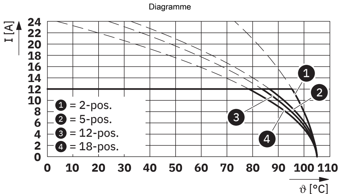
Type : FKCS 2,5/...-ST-5,08 avec FKIC 2,5/...-ST-5,08
