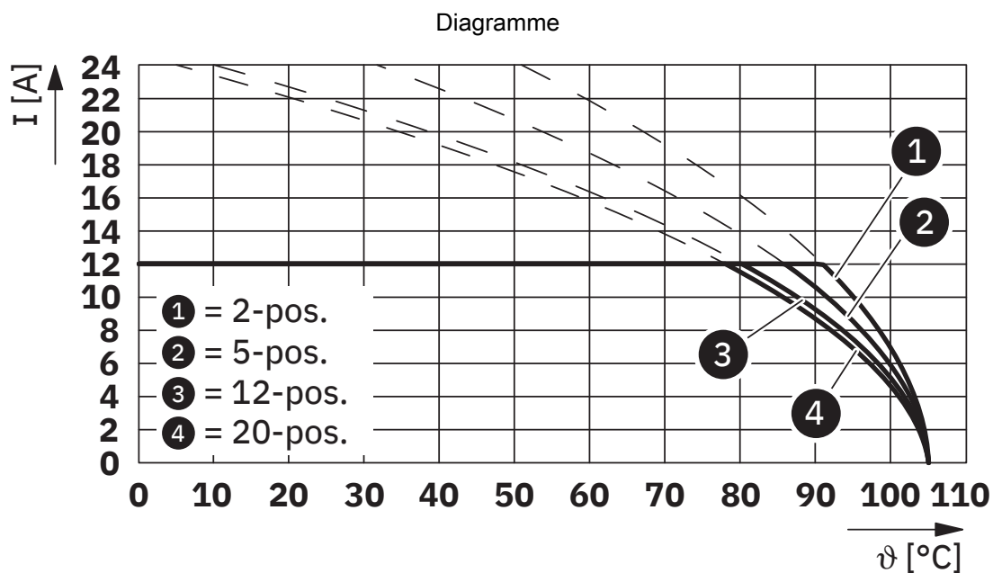
Type : FKCS 2,5/...-ST-5,08 avec IC 2,5/...-ST-5,08
