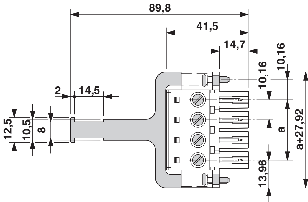
Dessin coté
