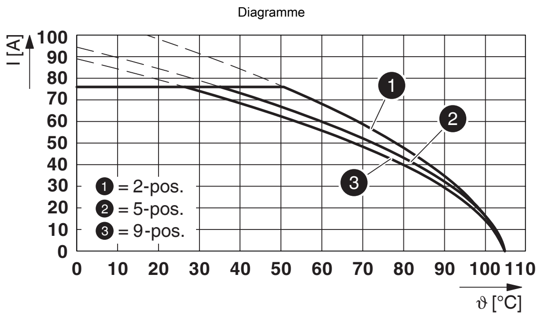
Type : PC 16/...-ST-10,16 avec ISPC 16/...-ST-10,16
