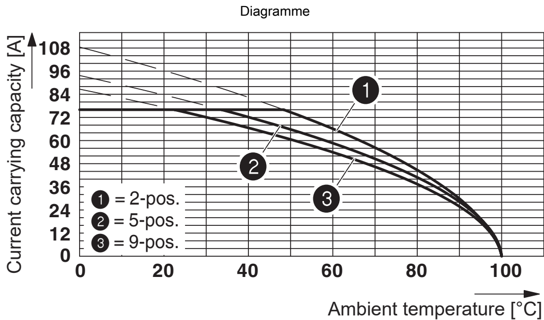
Courbe de derating pour : PC 16/...-ST-10,16 avec DFK-PC 16/...-ST-10,16
