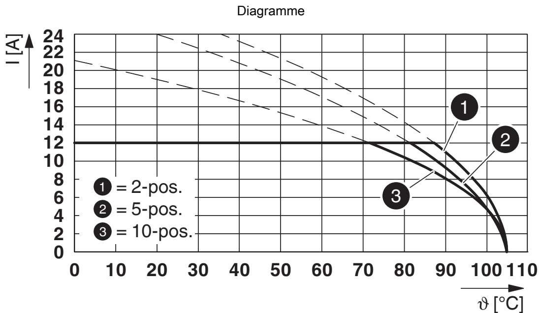
Type : TFKC 2,5/...-ST-5,08 avec SMSTBA 2,5/...-G-5,08
