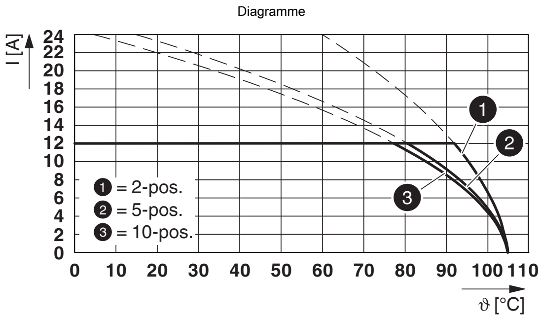
Type : TFKC 2,5/...-ST-5,08 avec SMSTB 2,5/...-G-5,08
