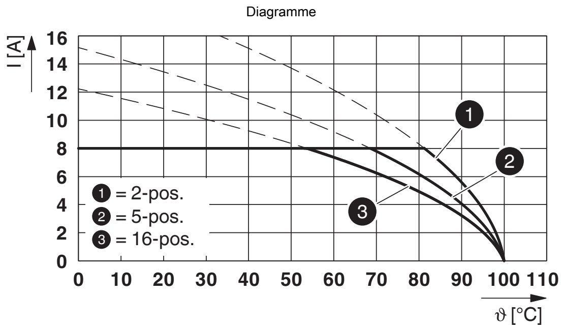
Type : FK-MCP 1,5/...-STF-3,81 avec MCD 1,5/...-GF-3,81
