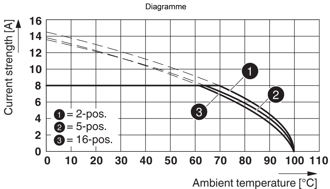
Type : FK-MCP 1,5/...-STF-3,81 avec DFK-MC 1,5/...-GF-3,81
