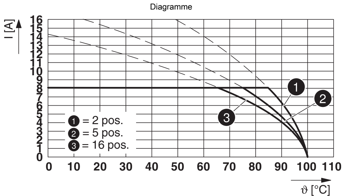
Type : FK-MCP 1,5/...-STF-3,81 avec MCDV 1,5/...-G1F-3,81
