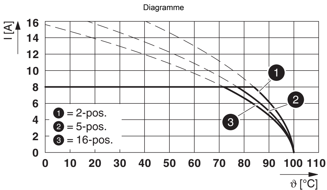
Type : FK-MCP 1,5/...-STF-3,81 avec IMC 1,5/...-STGF-3,81
