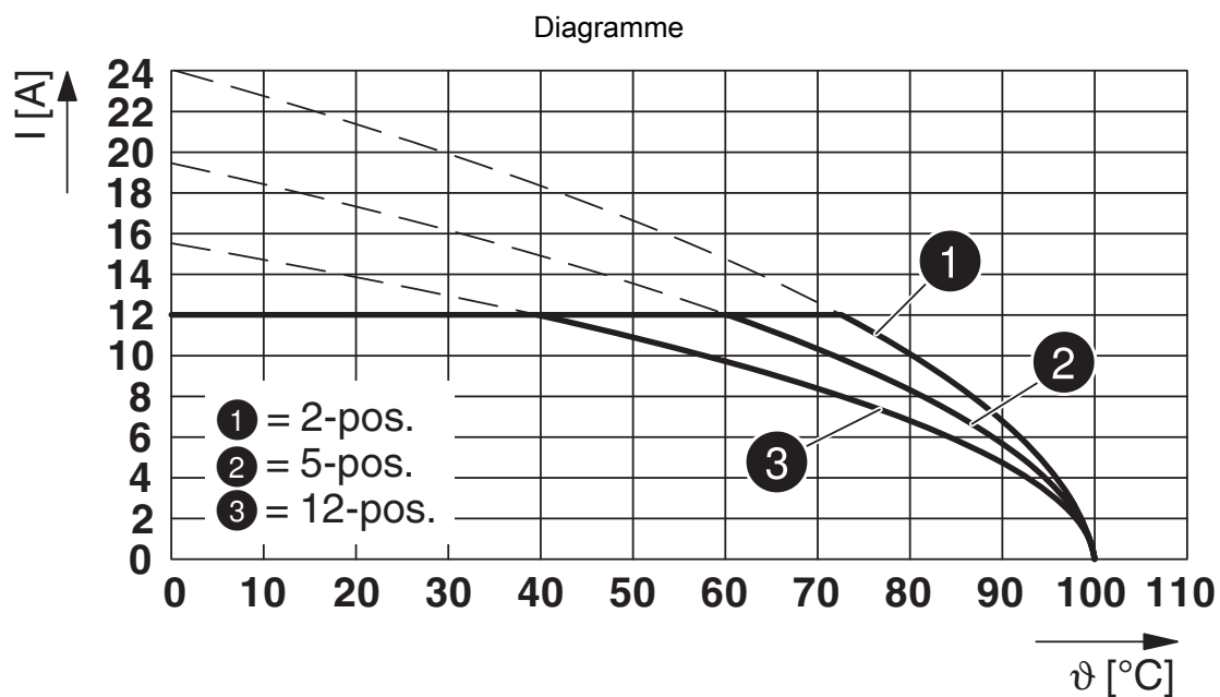
Type : MVSTB(R/W) 2,5/...-STF-5,08 avec CC 2,5/...-GF-5,08-LR P...THR
