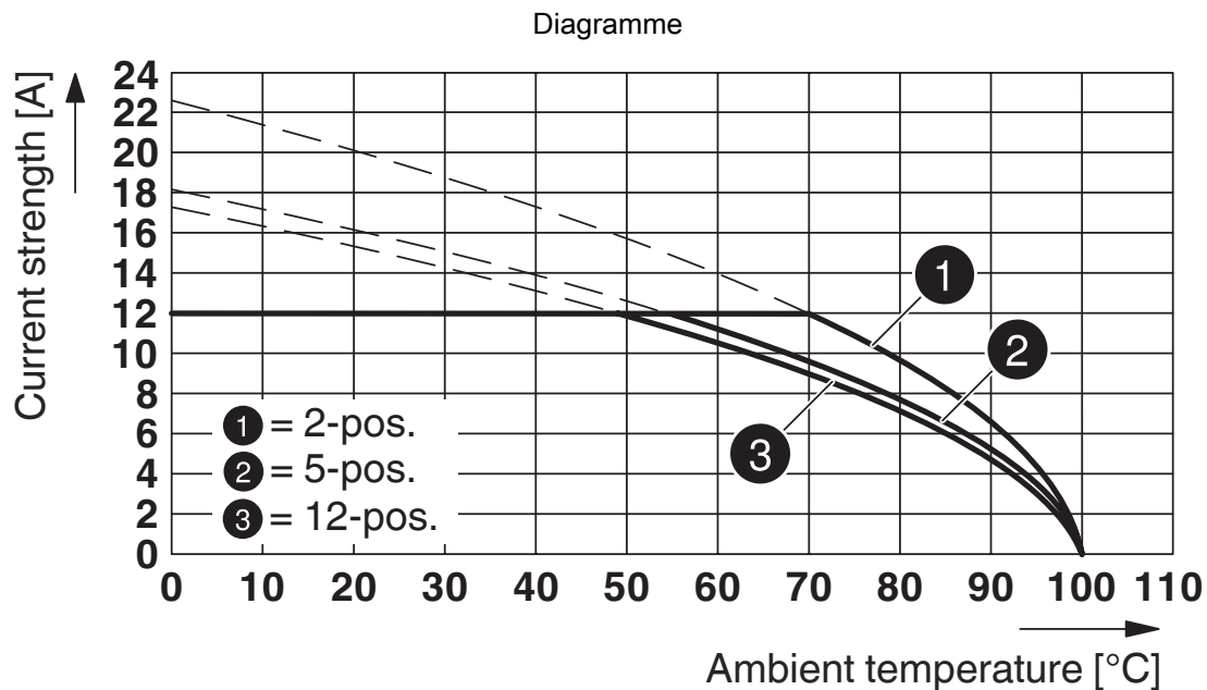
Type : MVSTB(R/W) 2,5/...-STF-5,08 avec CC 2,5/...-GF-5,08 P26THR
