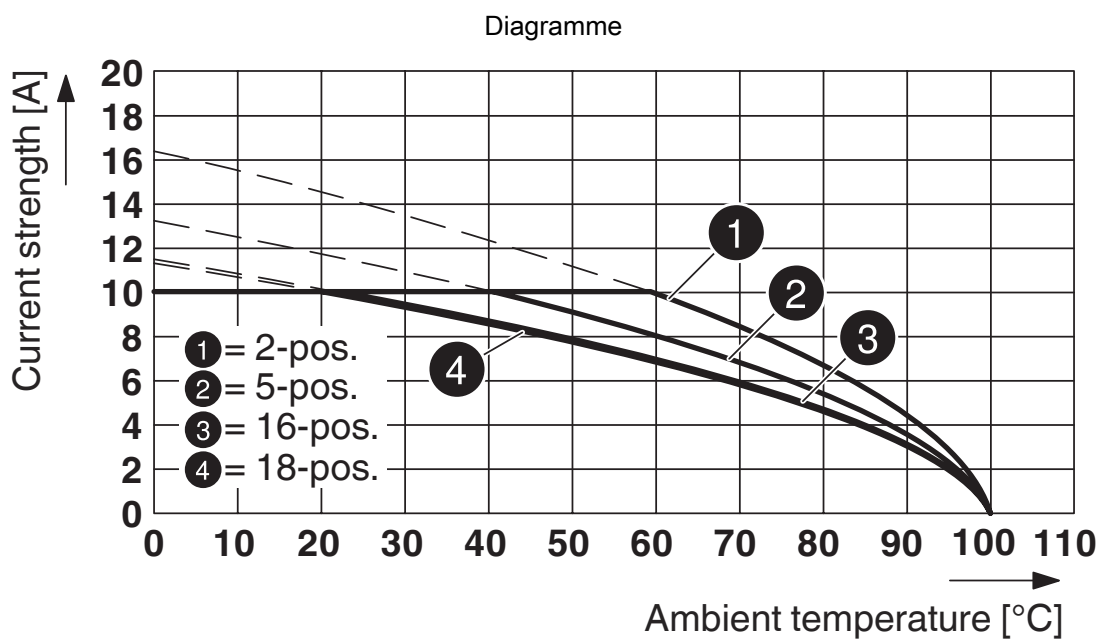
Type : MVSTB(R/W) 2,5/...-STF-5,08 avec MDSTBV 2,5/...-GF-5,08
