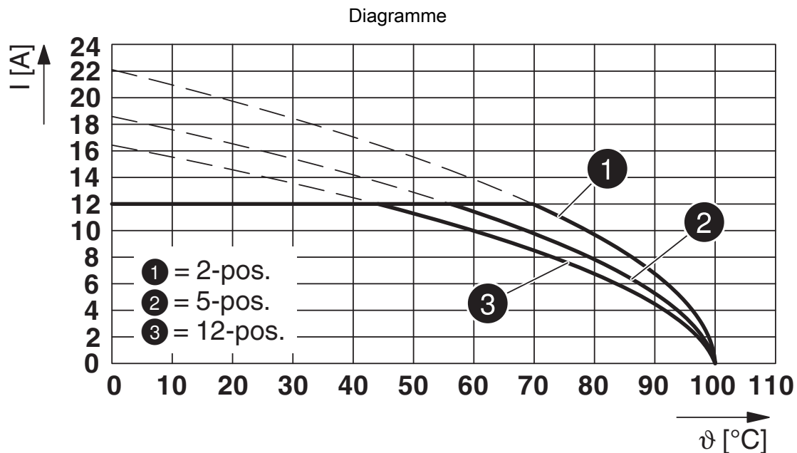
Type : MVSTB(R/W) 2,5/...-STF-5,08 avec CCV 2,5/...-GF-5,08-LR P...THR
