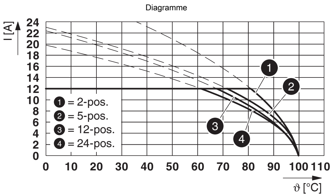
Type : IC 2,5/...-ST-5,08 avec ICV 2,5/...-G-5,08
