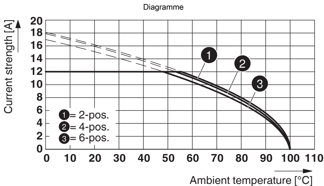
Type : GMVSTBW 2,5 HV/...-ST-7,62 avec GMSTBA 2,5/...-G-7,62
