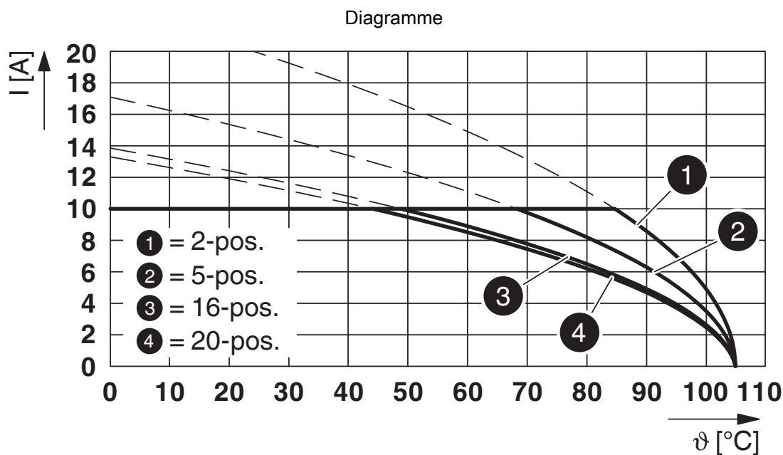
Type : IC 2,5/...-G-5,08 avec MDSTB 2,5/...-G1-5,08
