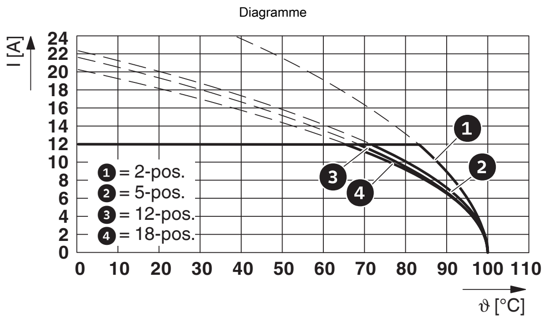
Type : MSTB 2,5/...-ST avec FKIC 2,5/...-ST
