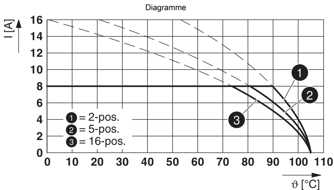
Type : FMC 1,5/...-STF-3,81 avec SMC 1,5/...-GF-3,81
