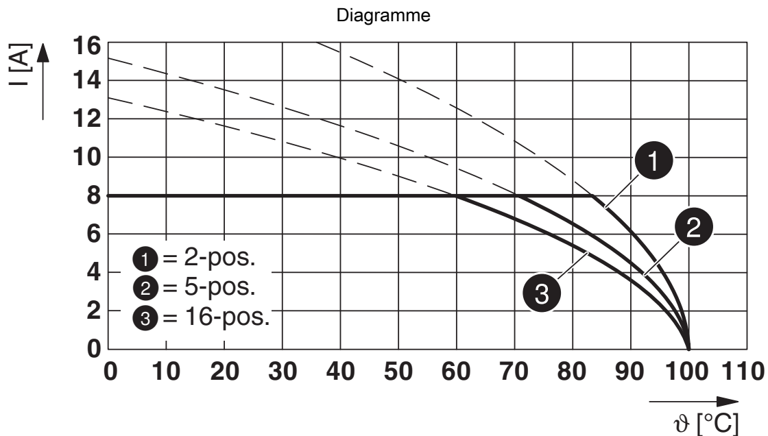
Type : FMC 1,5/...-STF-3,81 avec MCDV 1,5/...-GF-3,81
