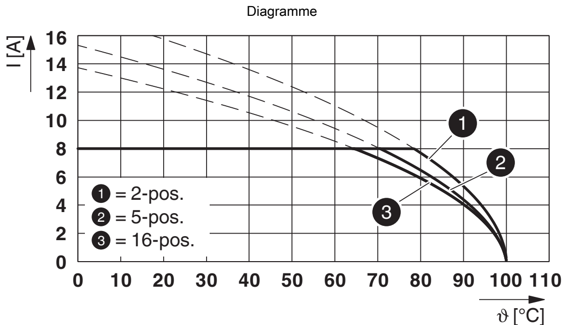
Type : FMC 1,5/...-STF-3,81 avec IMC 1,5/...-STGF-3,81
