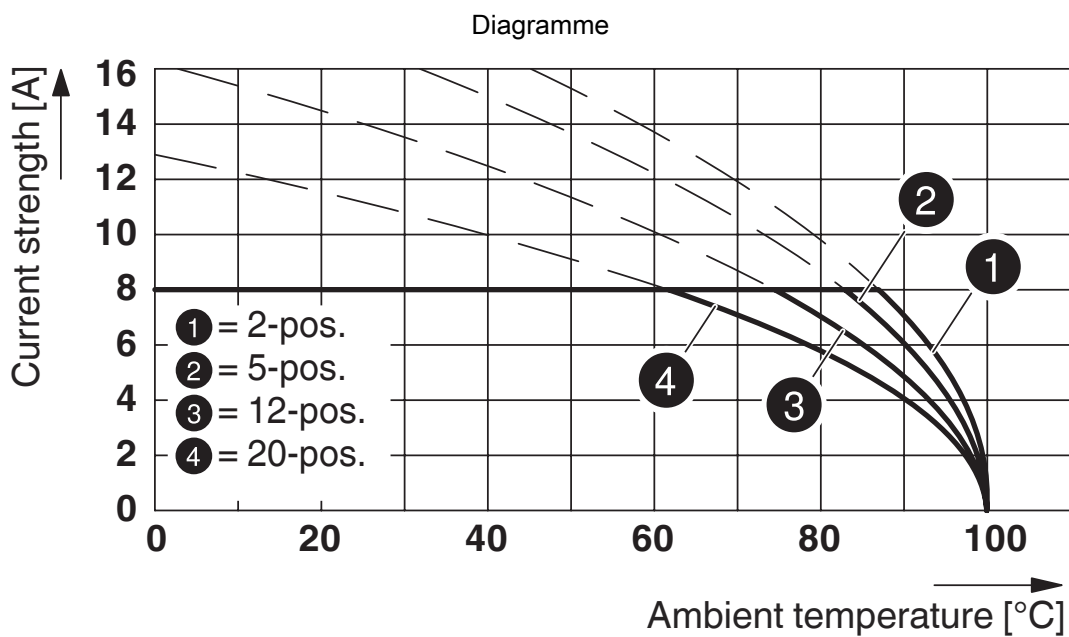
Type : FMC 1,5/...-STF-3,81 avec MCV 1,5/...-GF-3,81 P... THR
