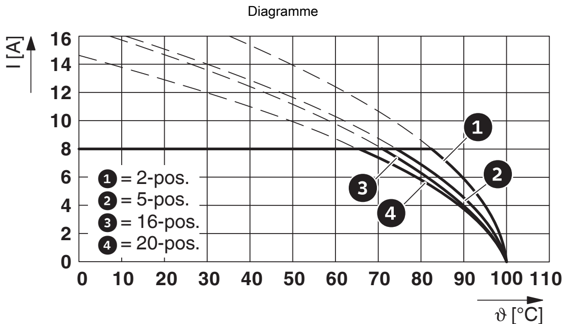
Type : FMC 1,5/...-STF-3,81 avec MC 1,5/...-GF-3,81 P...THR
