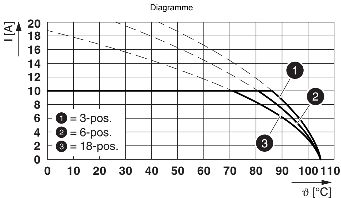
Type : FKCN 2,5/...-ST avec MDSTBV 2,5/...-G1
