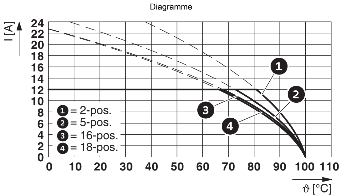
Type : FKCN 2,5/...-ST avec MSTBW 2,5/...-G
