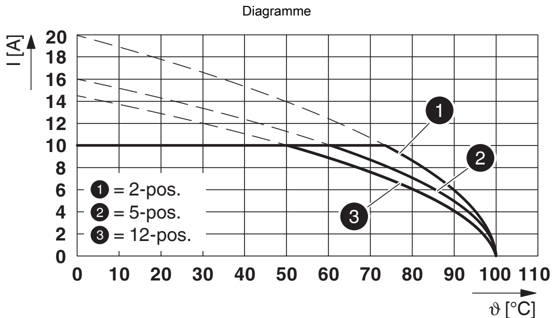
Type : FKCN 2,5/...-ST avec MDSTBVA 2,5/...-G
