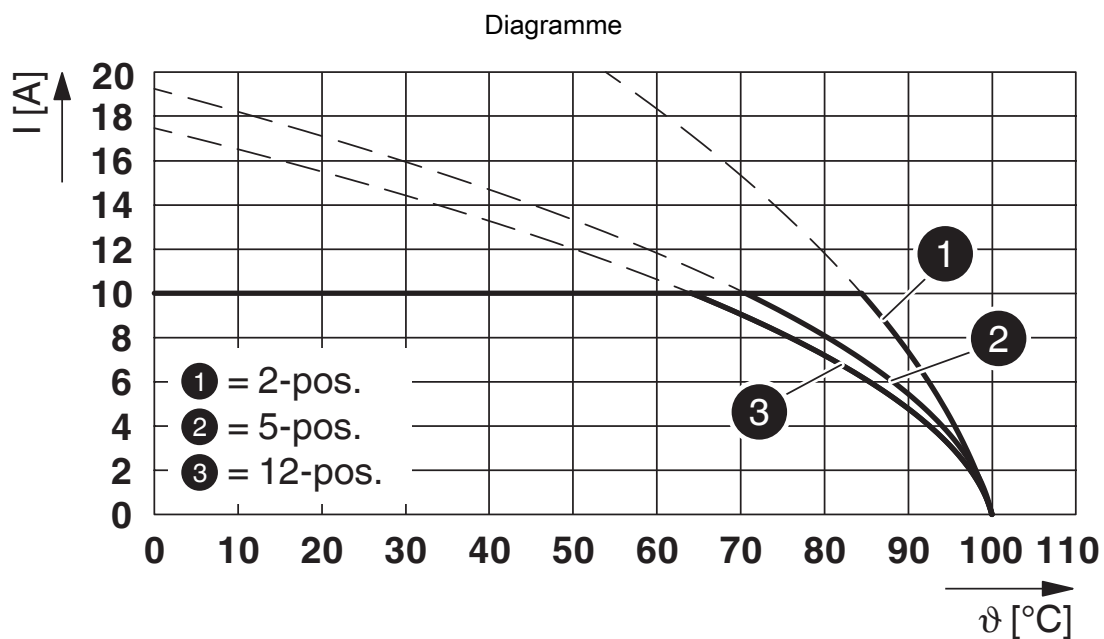
Type : FKCN 2,5/...-ST avec MDSTBW 2,5/...-G
