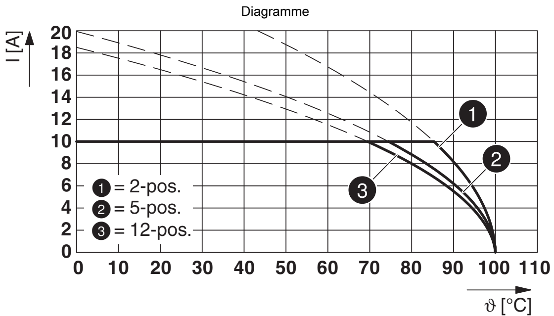
Type : FKCN 2,5/...-ST avec MDSTB 2,5/...-G
