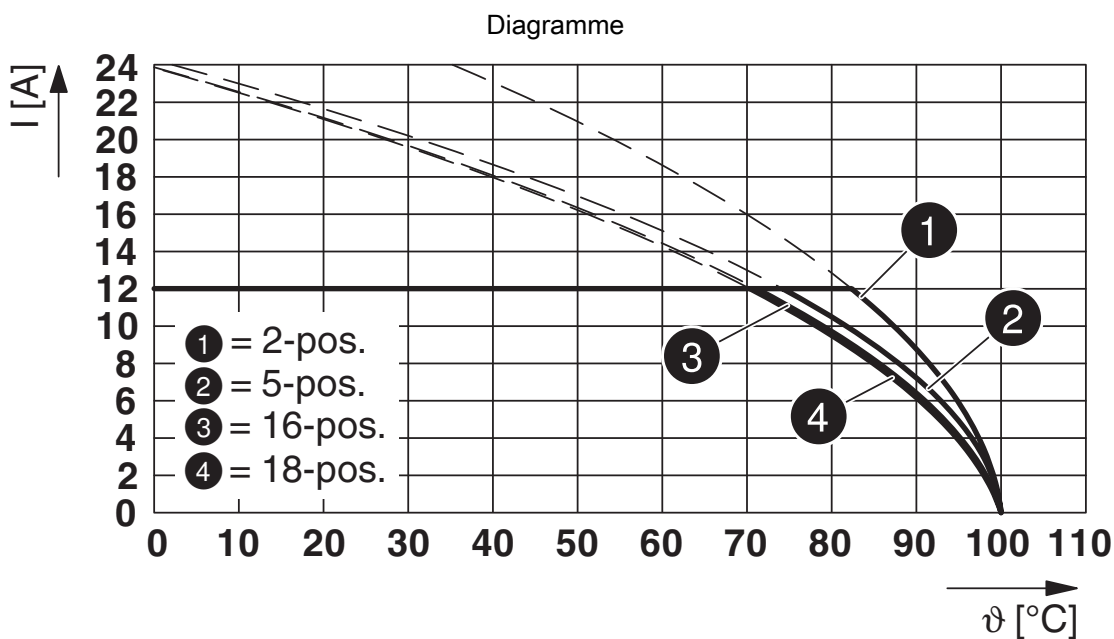
Type : FKCN 2,5/...-ST avec SMSTBA 2,5/...-G
