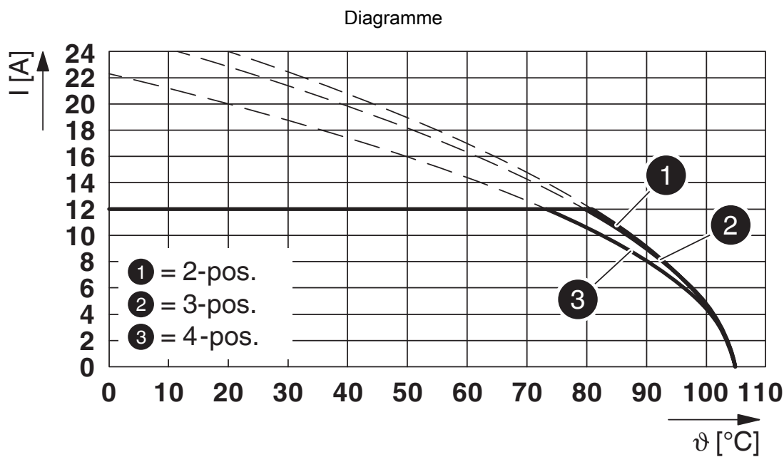
Type : FKCN 2,5/...-ST avec MSTBO 2,5/...-G1R
