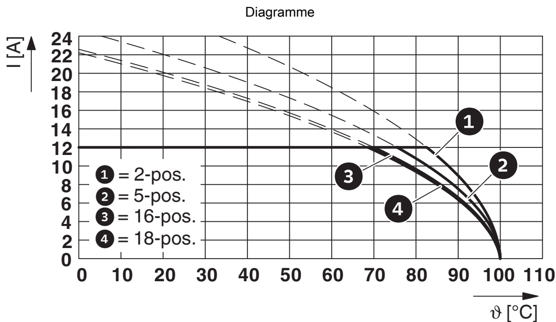
Type : FKCN 2,5/...-ST avec SMSTB 2,5/...-G
