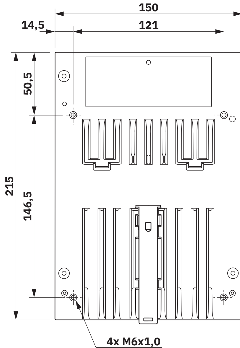
Dessin coté
