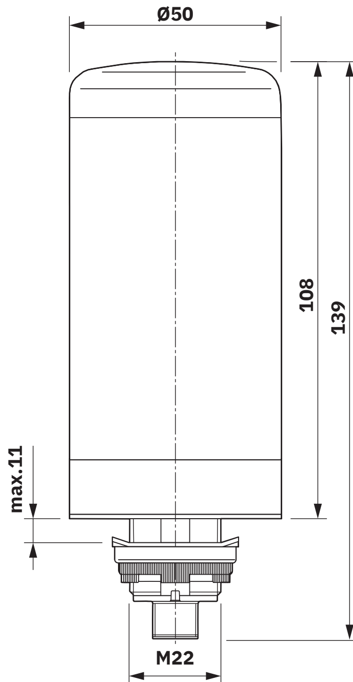
Dessin coté
