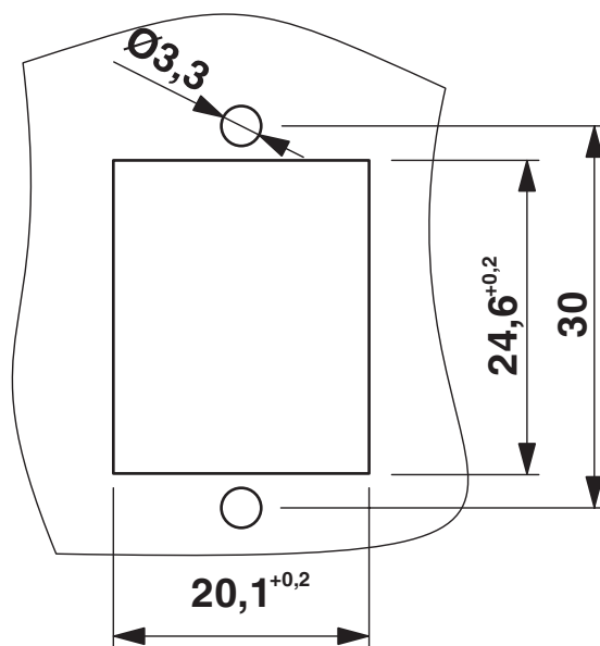
Dessin coté
