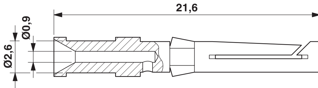
Dessin coté
