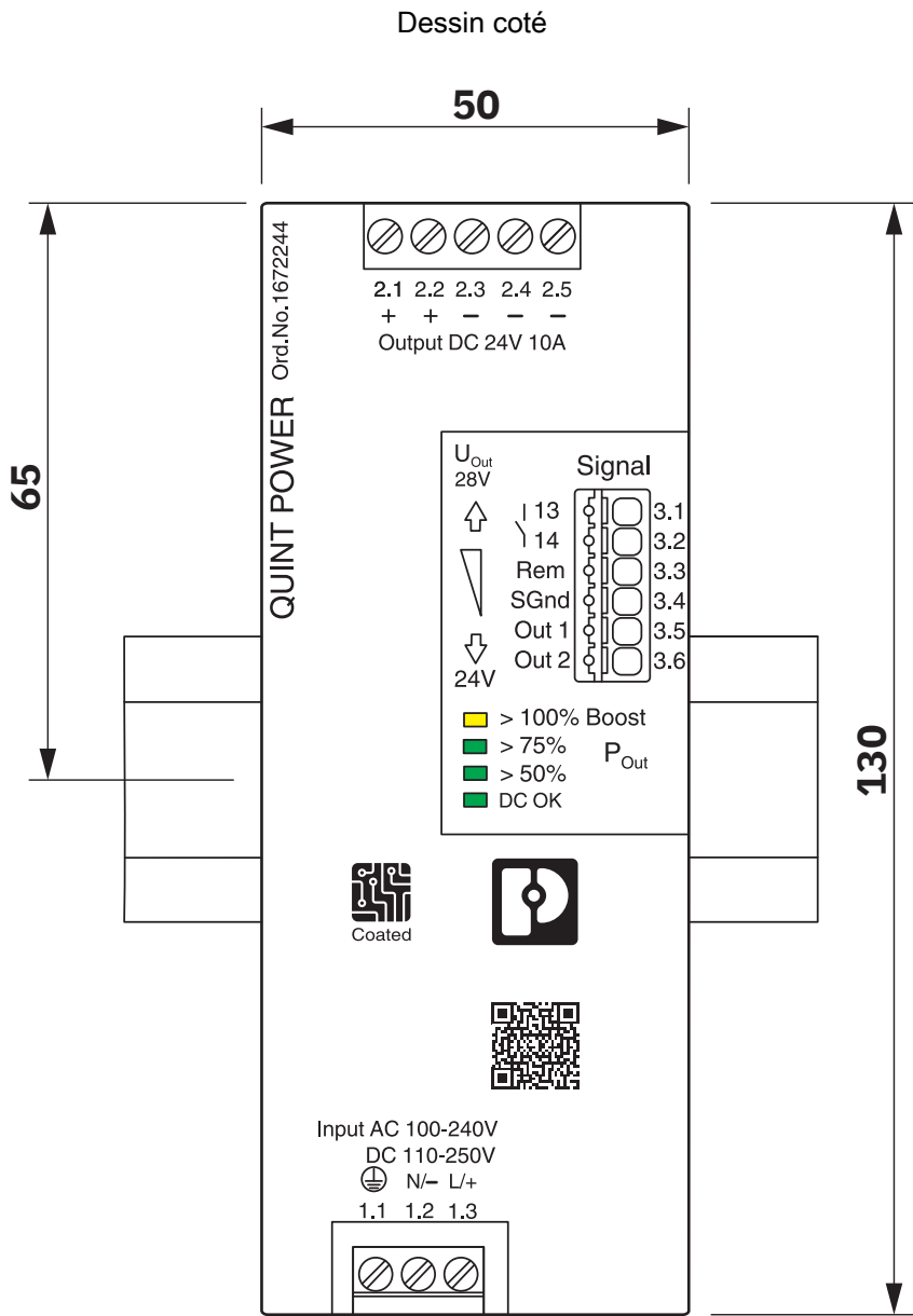
Encombrement de l'appareil (cotes en mm)
