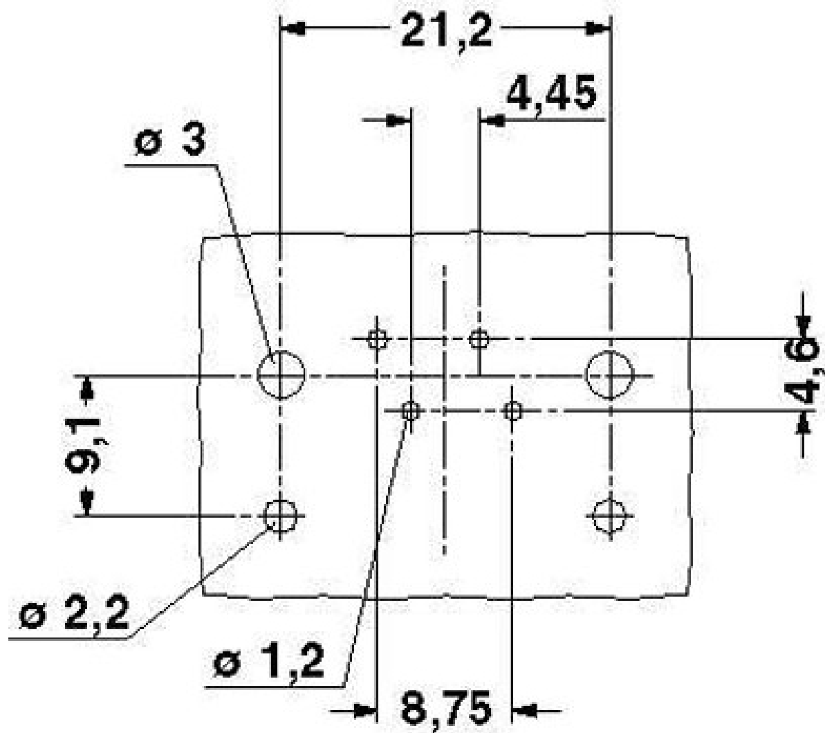
Gabarit perçage / géom. pastille soudage
