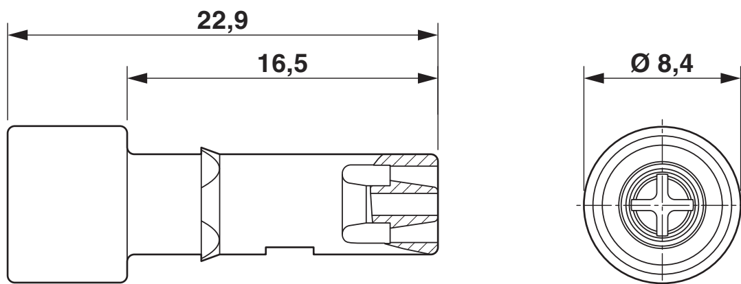
Dessin coté
