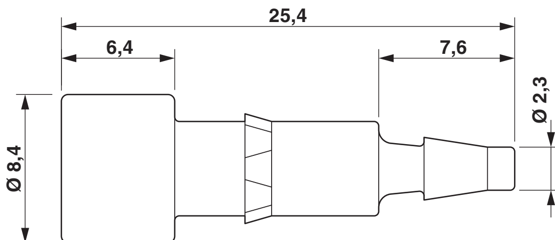
Dessin coté
