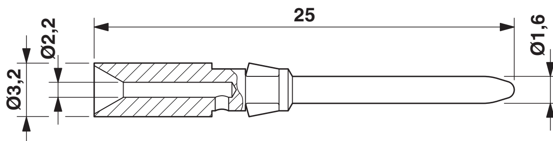
Dessin coté
