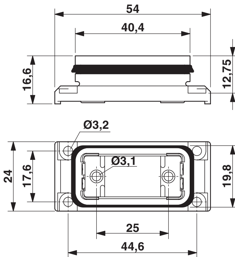
Dessin coté
