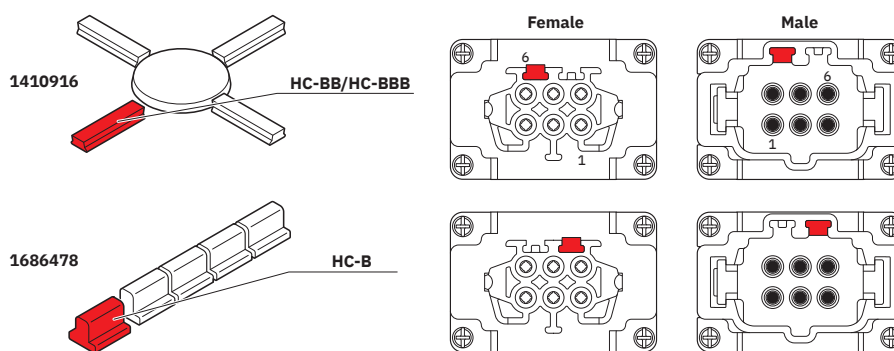
Dessin schématique
