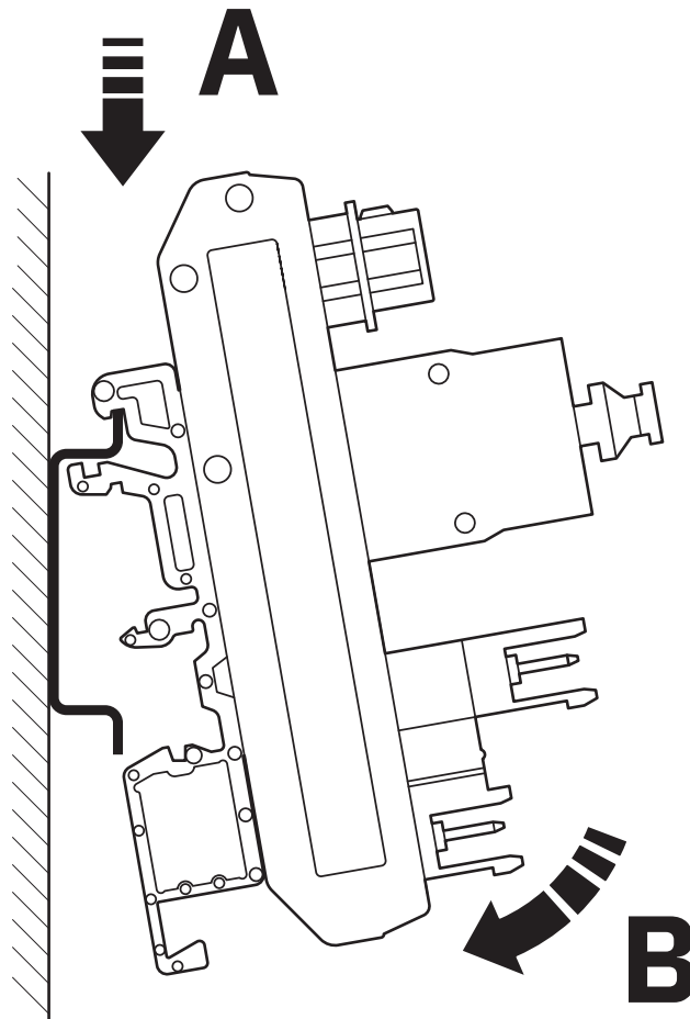
Dessin schématique
