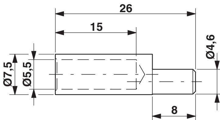
Dessin coté
