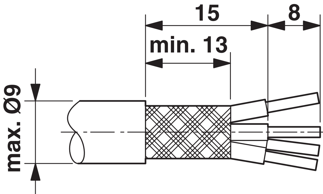
Dessin coté
