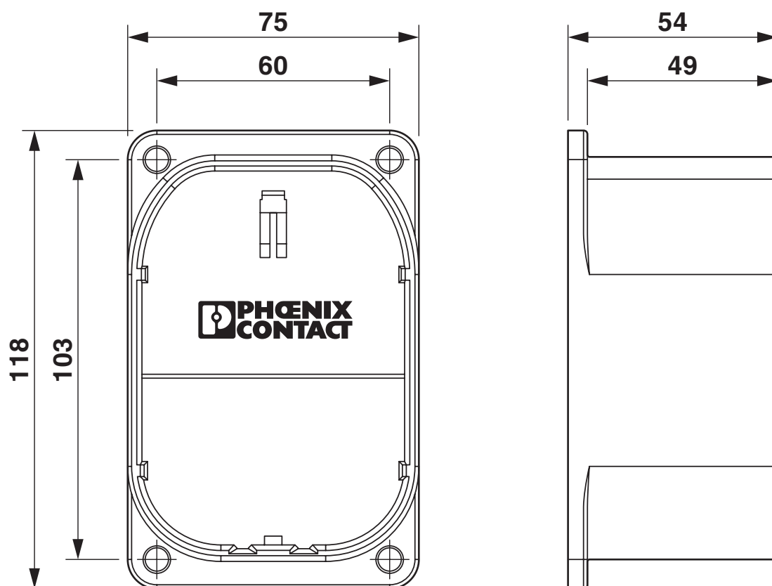
Dessin coté
